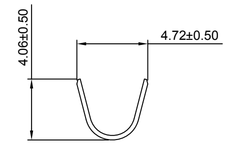
SEC:A-A
