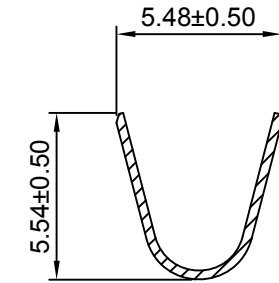
SEC:A-A
